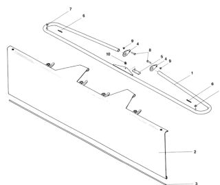
ETB-011499, Dociskacz
