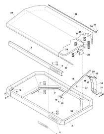
ETB-011495, Nadstawka nad zbiornik ze składaną planką L
