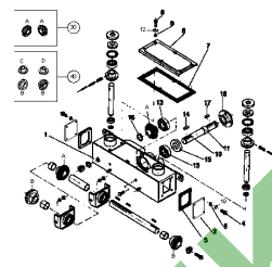
ETB-011485, Przekładnia (1/2)
