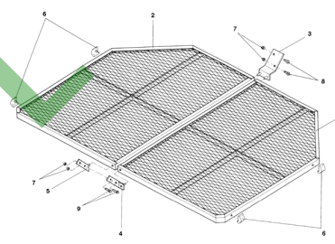
ETB-011498, Sito chroniące przed ciałami obcymi, składane
