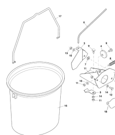
ETB-011497, Urządzenie do ustawiania odpowiedniej dawki rozsiewu
