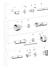
ETB-011493, Wałek przełącznikowy ze sprzęgłem ciernym, 710 mm
