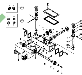
ETB-011486, Przekładnia (2/2)
