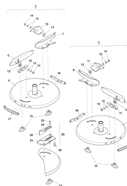
ETB-011487, Tarcze rozsiewające
