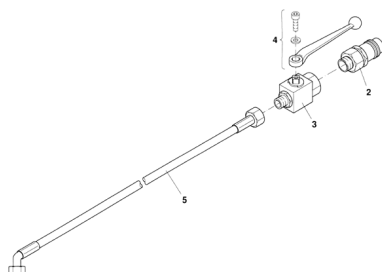
ETB-011491, Wąż hydr. do sterowania indywidualnego
