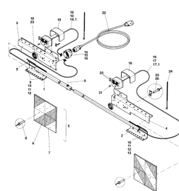
ETB-011500, Instalacja oświetleniowa
