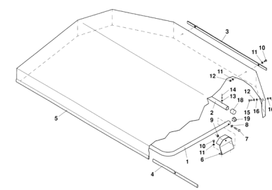
ETB-011494, Składana plandeka N
