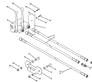
ETB-011490, Zespół dwudrogowy
