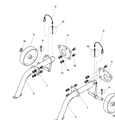
ETB-011502, Kółka transportowe, składane
